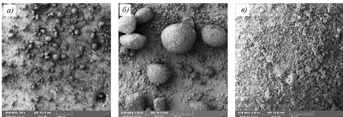
Рис. 1. Микроструктура ( \times 200 (a), \times 1000 (б) и \times 6000 (в)) порошка \text{Al}_2\text{O}_3 , используемого для приготовления керамических композиций
