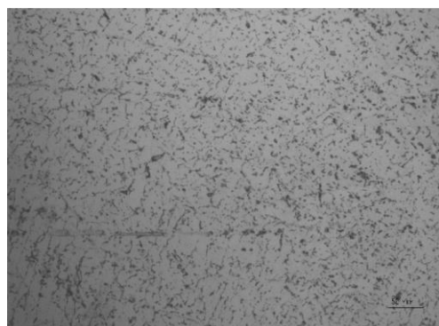
Рис. 12. Микроструктуры ( \times 50 ) наплавленного образца, выполненного лазерной сваркой
